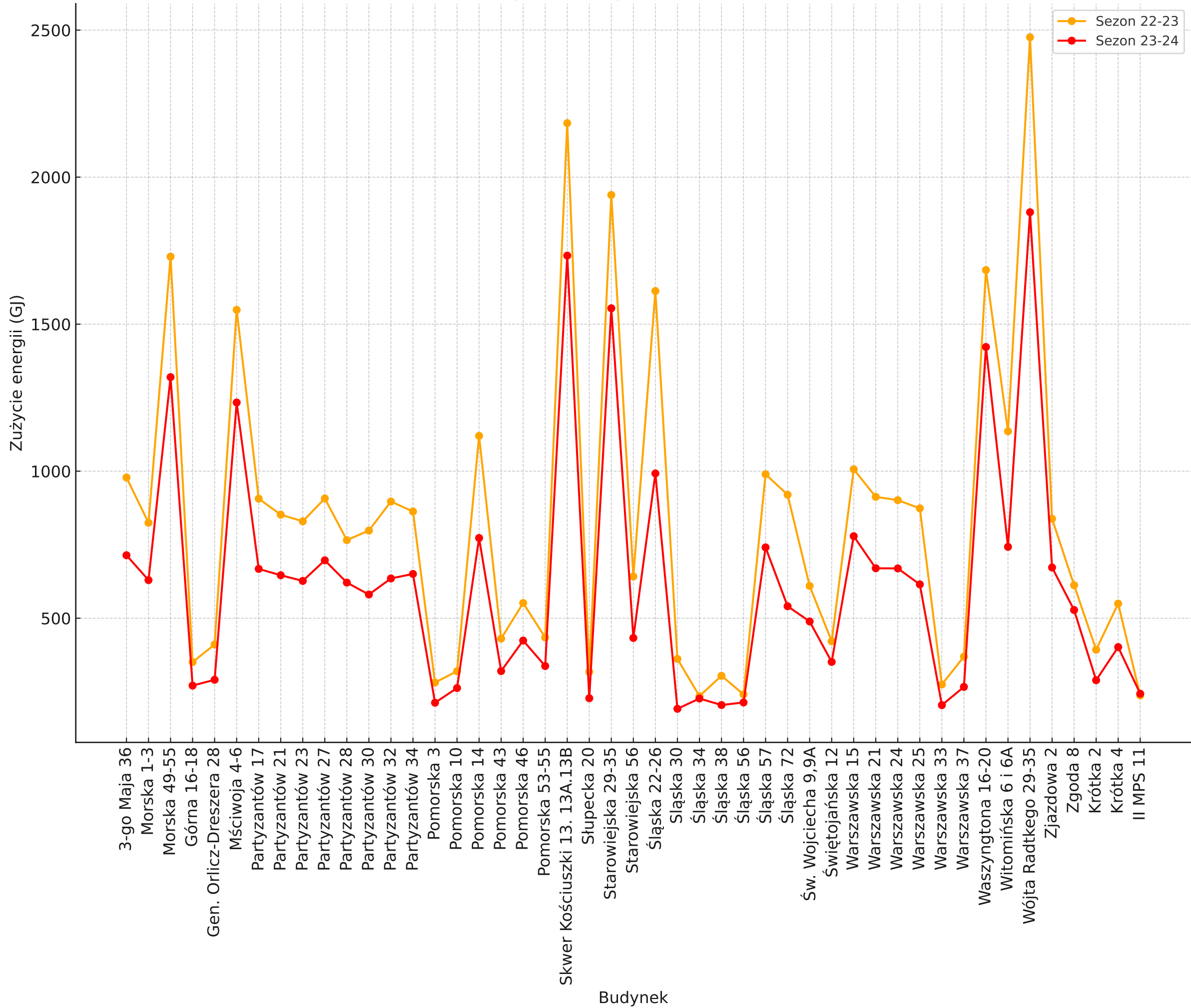
Porównanie zużycia energii w sezonach 22-23 i 23-24
